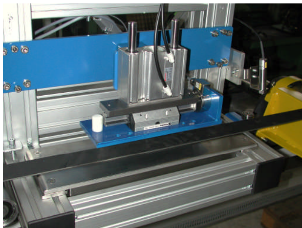
Riemen-Prüfstand mit Pneumatischer Anpressvorrichtung
