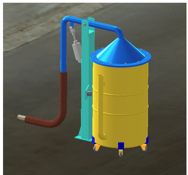
Fasskühlstation, Deckel mit Pneumatikzylinder anhebbar
